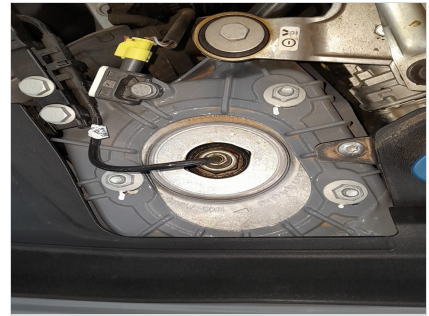
TORRE DO AMORTECEDOR ESQUERDA
